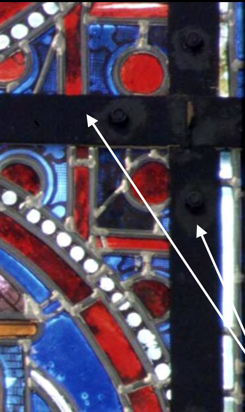
Izgled armature iz unutrašnjosti, Laon katedrala.
